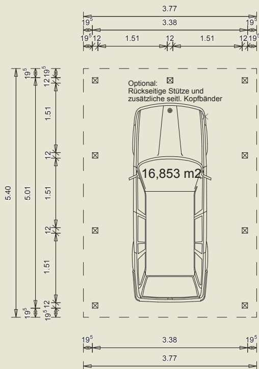
GRUNDRISS
