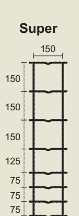
Höhe 80 cm Typ 80/8
