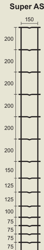
Höhe 200 cm Typ 200/15
