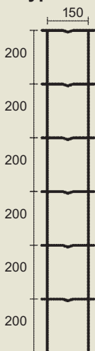
Höhe 120 cm Typ 120/7
