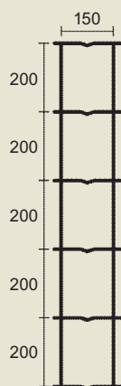
Höhe 100 cm Typ 100/6
