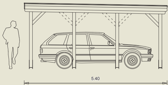
SEITENANSICHT
