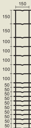
Höhe 130 cm Typ 130/18
