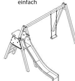
701510 Schaukel-Rutsche Kombi einfach
