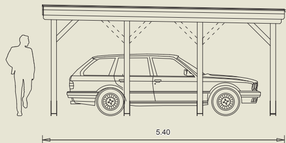
Optionale Stütze und Kopfbänder
