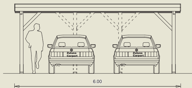
VORDERANSICHT
