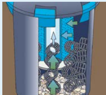
▲ Filtermaterialien Bio-Filterflächen, mit der speziell entwickelten Strömungsführung, bieten neben den Filterschwämmen noch einmal zusätzliche Besiedelungsfläche für Filterorganismen und befinden sich frei beweglich im Wasserstrom.
