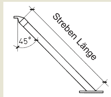
Platte 10 x 10 cm 2 Löcher Ø 12 mm
