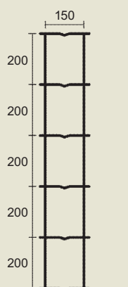
Höhe 100 cm Typ 100/6
