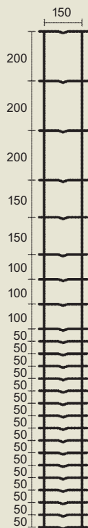
Höhe 200 cm Typ 200/25 MEDIUM
