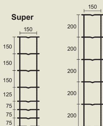
Höhe 80 cm Typ 80/8
