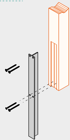
T-Eisen im Pfosten eingelassen
