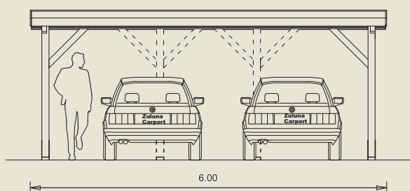
VORDERANSICHT
