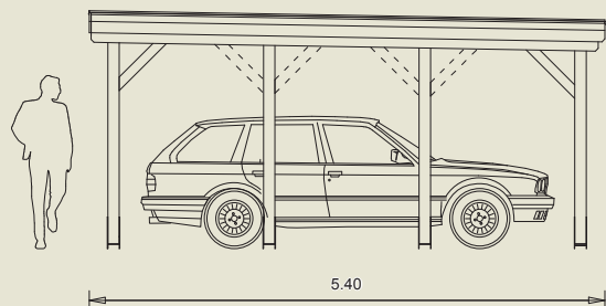
SEITENANSICHT
