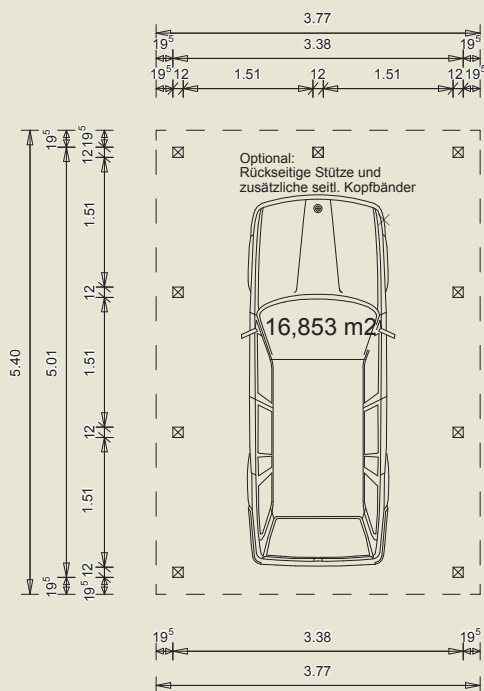
GRUNDRISS
