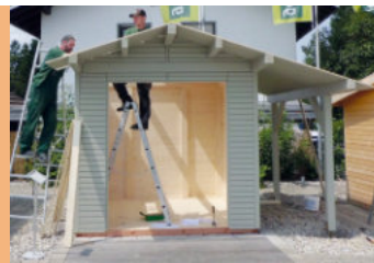
Erstellung der Dachschalung
