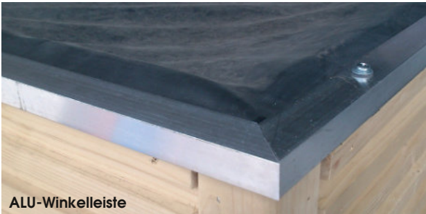
Optionale Blehabdeckungsvarianten
