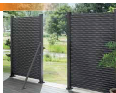
GLAS im Design Klar kombiniert mit FLOW, Klemmpfosten und Sturmkanker als Zusatzsicherung in Anthrazit.
